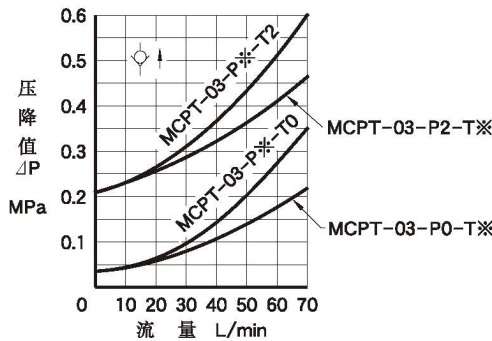
自由流压降特性
