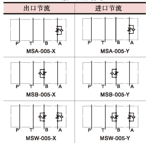
JIS液压图形符号
