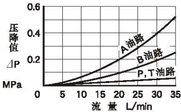
压降特性
