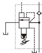
JIS液压图形符号
