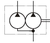
JIS液压图形符号
